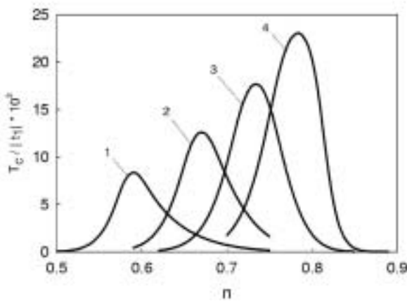
Рис. 1. Влияние перескоков в третью координационную сферу на концентрационную зависимость T_c при различных \alpha_3 = t_3/t_1 : 1) \alpha_3 = 0 ; 2) \alpha_3 = -0,1 ; 3) \alpha_3 = -0,2 ; 4) \alpha_3 = -0,3 . Параметры модели: t_2/t_1 = -0,2 , |t_1|/U = 0,2
